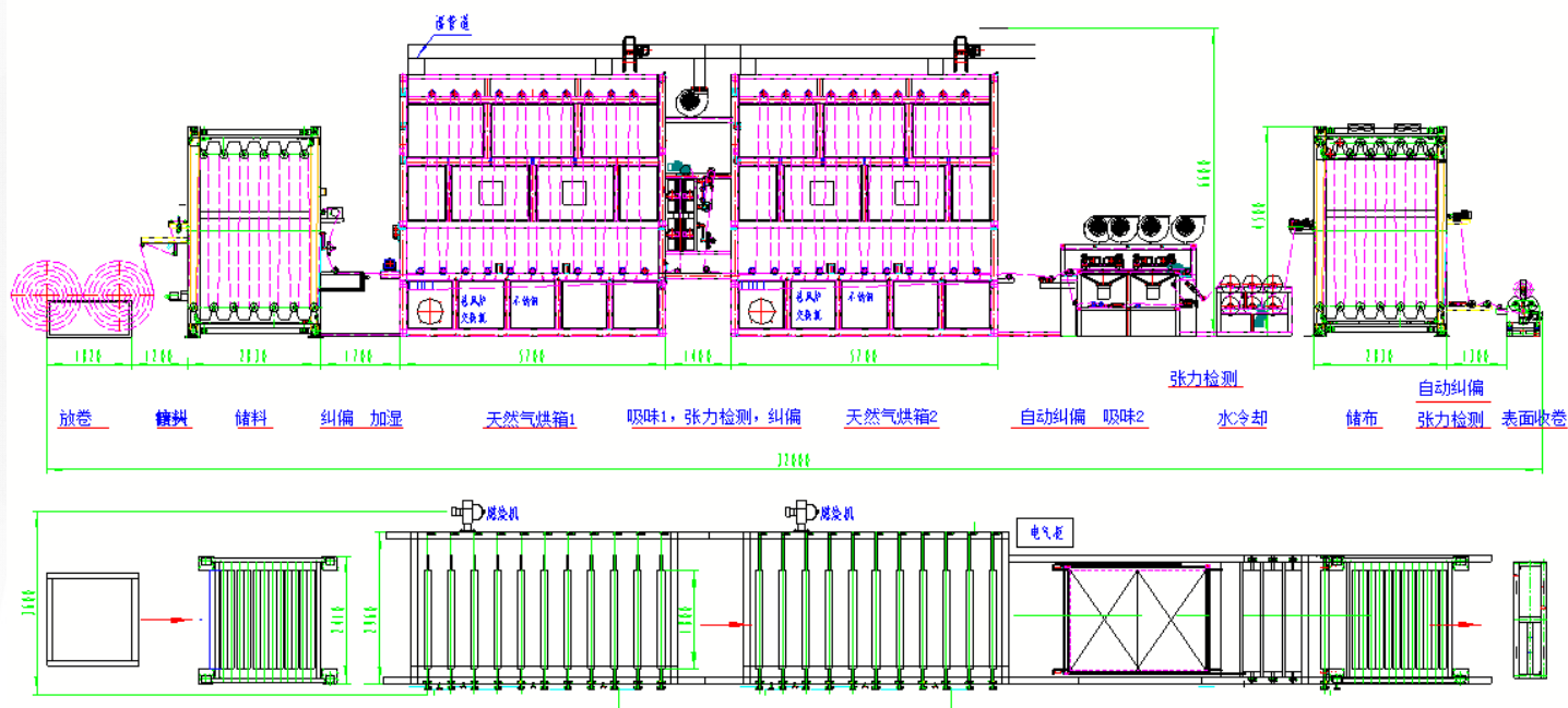
HY-2000CWA型 内置加热式立式除味机示意图
